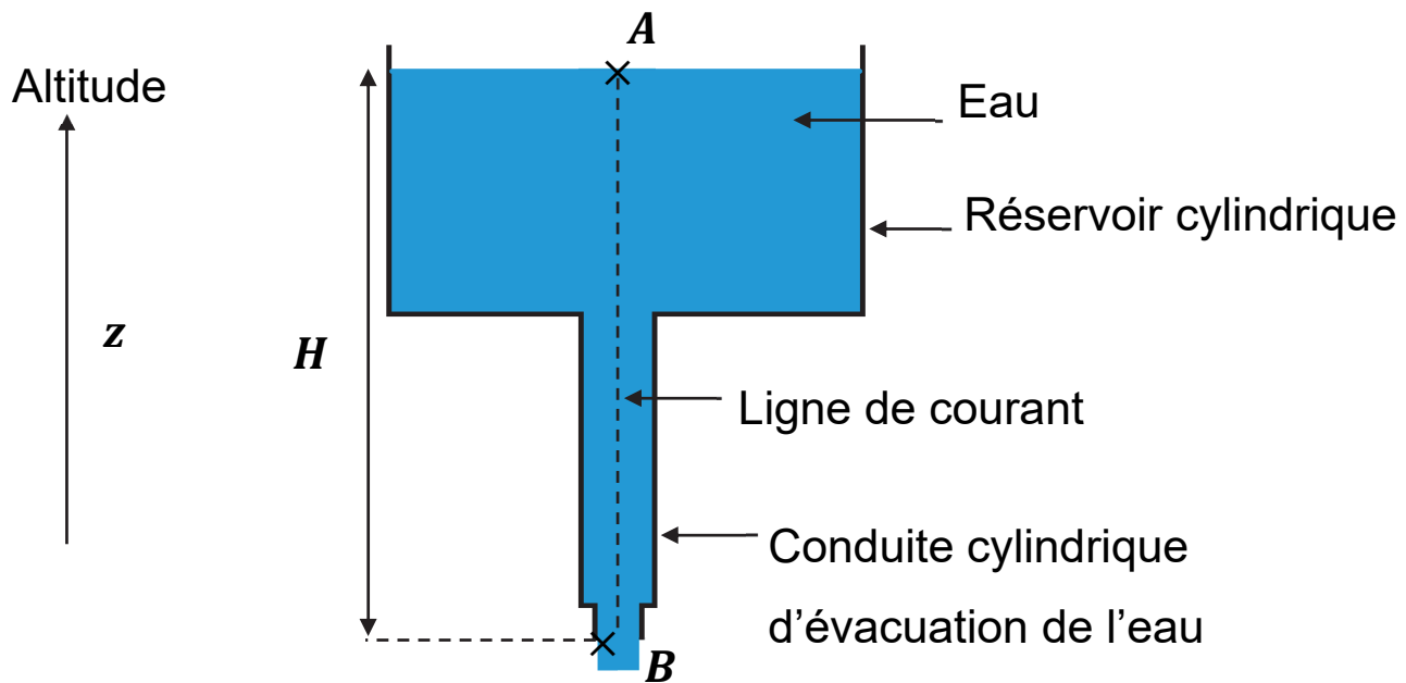
Figure 2. Schéma de principe du réservoir d'eau embarqué dans le dirigeable.
