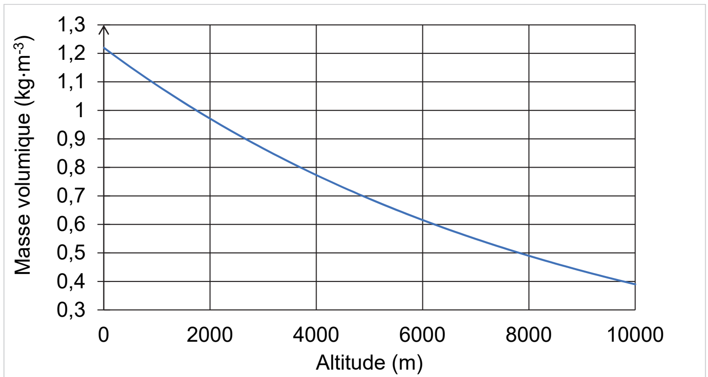
Figure 1. Représentation de l'évolution de la masse volumique de l'air en fonction de l'altitude
